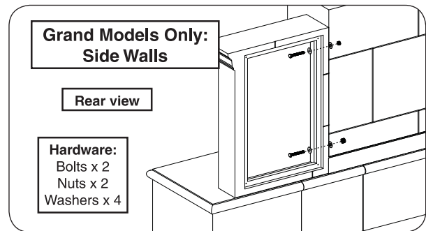
Fig. 19-1 Assemble side-wall (skip if n/a)
