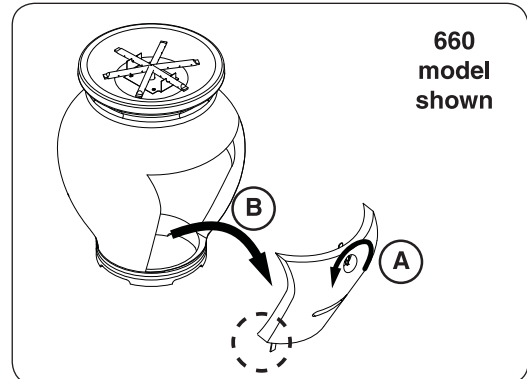
Fig. 15-1 Remove storage door (Amphora)
