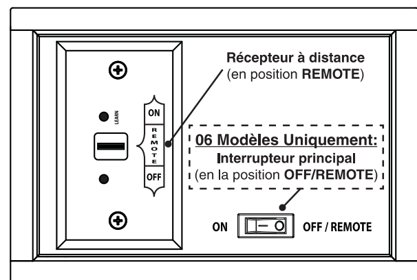
Fig. 30-1 Contrôle détail du panneau
