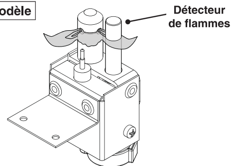
Fig. 32-2 Bonne flamme pilote
