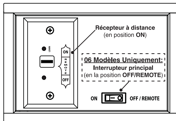
Fig. 40-1 Contrôle détail du panneau
