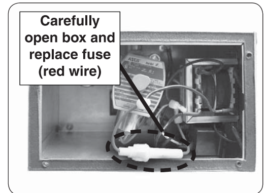
Fig. 42-3 Replace fuse
