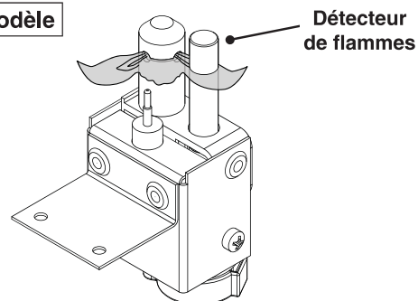
Fig. 38-2 Bonne flamme pilote
