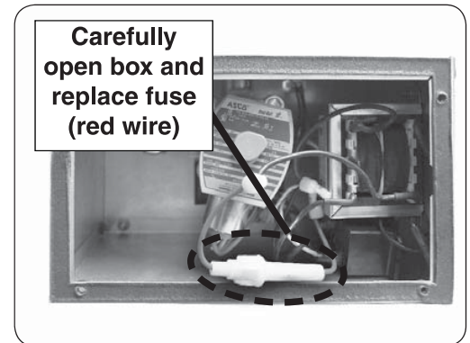
Fig. 40-3 Replace fuse
